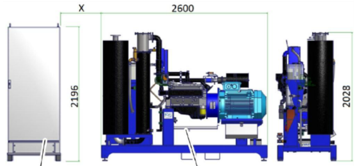
40 KW system med gen gas generator och generator.
